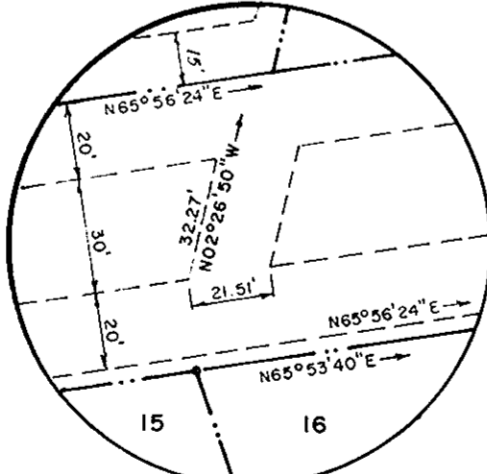
INSERT "A" SCALE: 1" = 50'
