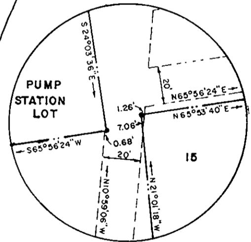
INSERT "C" SCALE: 1" = 50'
